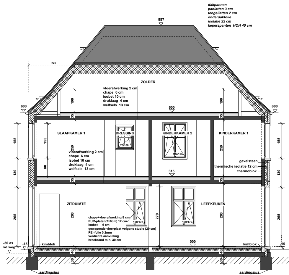
DOORSNEDE AB 1/100
