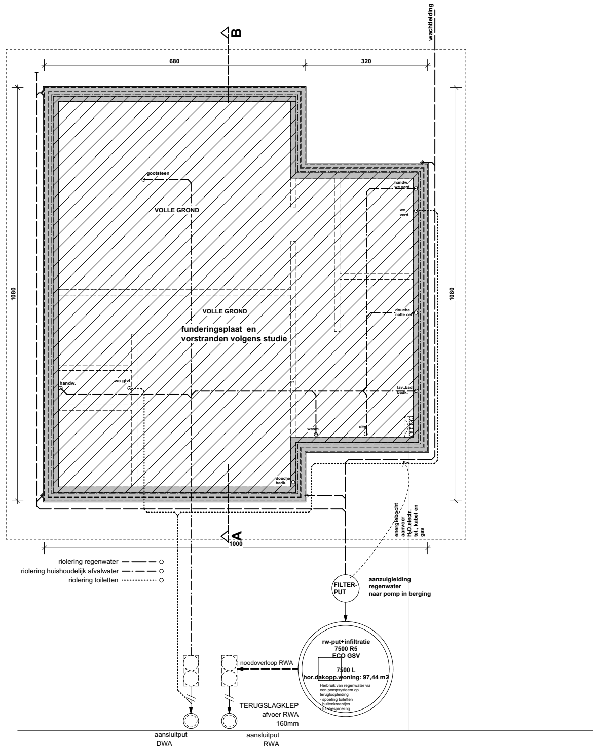
FUNDERINGS-en RIOLERINGSPLAN 1/100 NR 61
